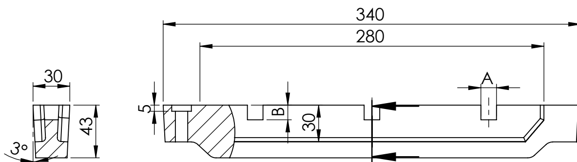
SEÇÃO - ESCALA 1 : 3
