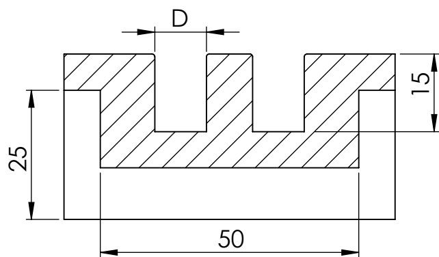
SEÇÃO A-A
