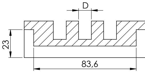
SEÇÃO A-A ESCALA 1 : 1.5
