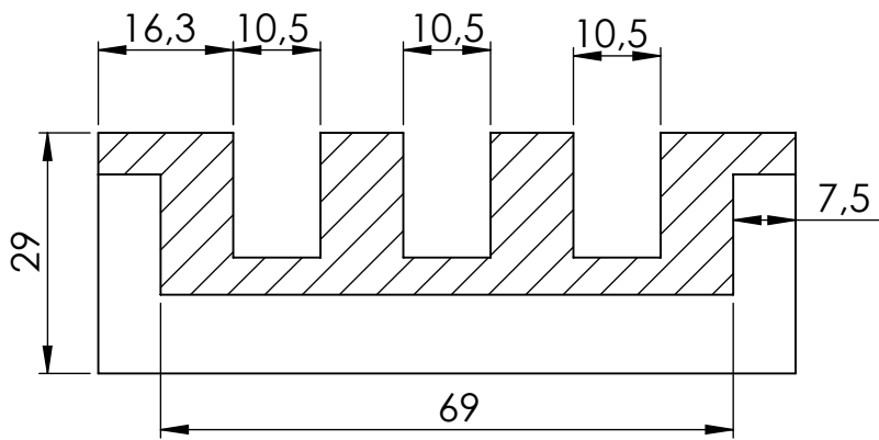
SEÇÃO A-A ESCALA 1 : 1
