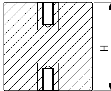
SEÇÃO A-A
